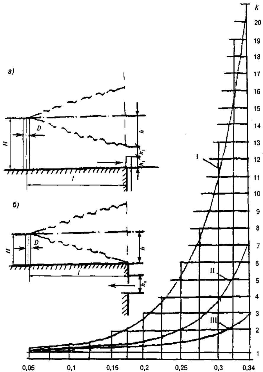
а - расположение источника над зоной всасывания наружного воздуха приемным устройством (высота трубы источника H = 2h_1 + h ); б- то же, над кровлей здания (высота трубы источника H = h ); h - расстояние по вертикали, м, горизонтальной оси струи; h_1 , - высота отверстия для приема наружного воздуха, м; l - расстояние между устьем источника и приемным устройством для наружного воздуха, м.
